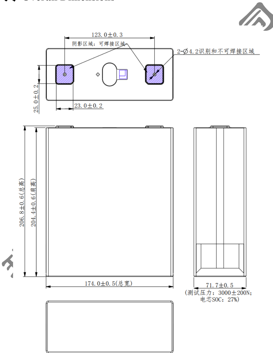
Figure 7 电池尺寸 /mm
